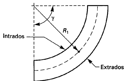
FIG. 304.2.1 NOMENCLATURE FOR PIPE BENDS
