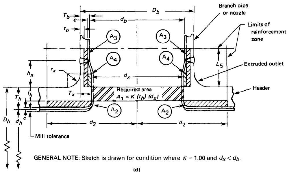
FIG. 304.3.4 EXTRUDED OUTLET HEADER NOMENCLATURE (CONT'D)
